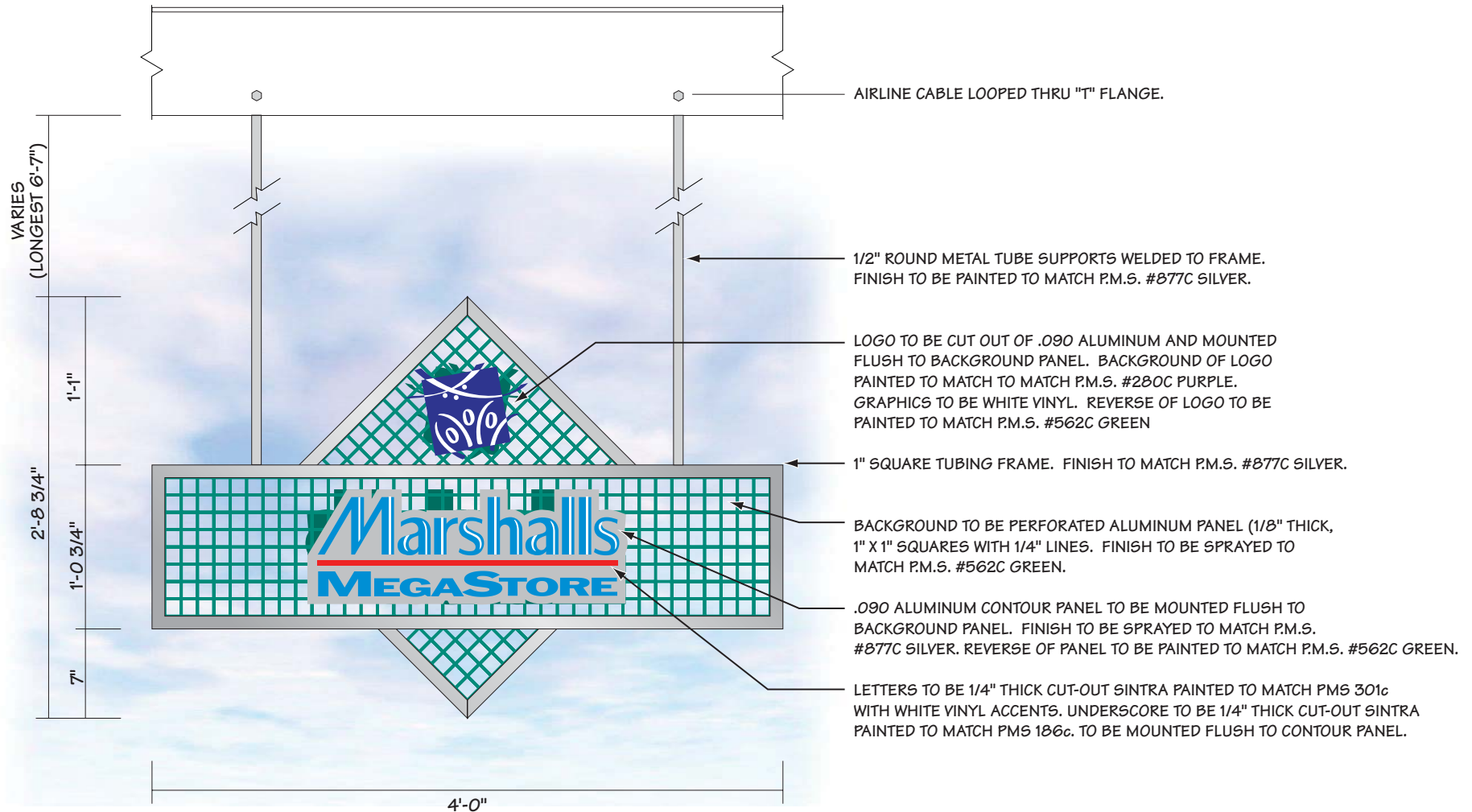
1. Blade Sign Panel SCALE: 1" = 1'-0"
