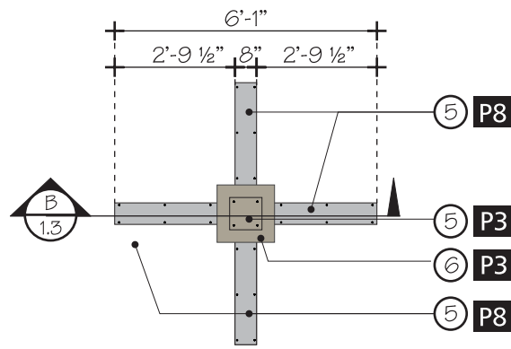
1 TOP VIEW SCALE: 1/4" = 1'-0"
